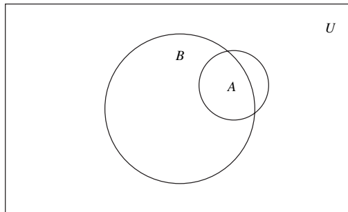
FIGURA A-2 Diagrama de Venn para representar A \not\subset B
