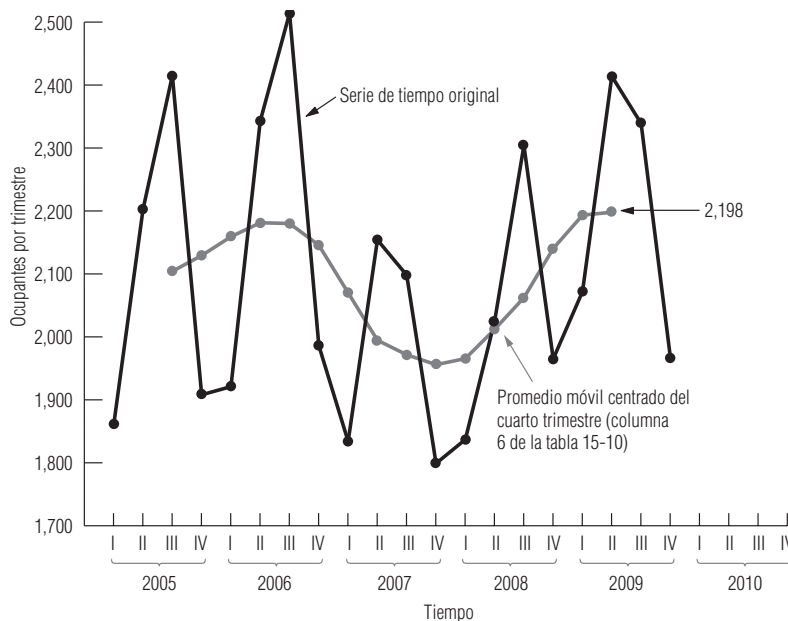
FIGURA 15-7 Uso de un promedio móvil para suavizar la serie de tiempo original
