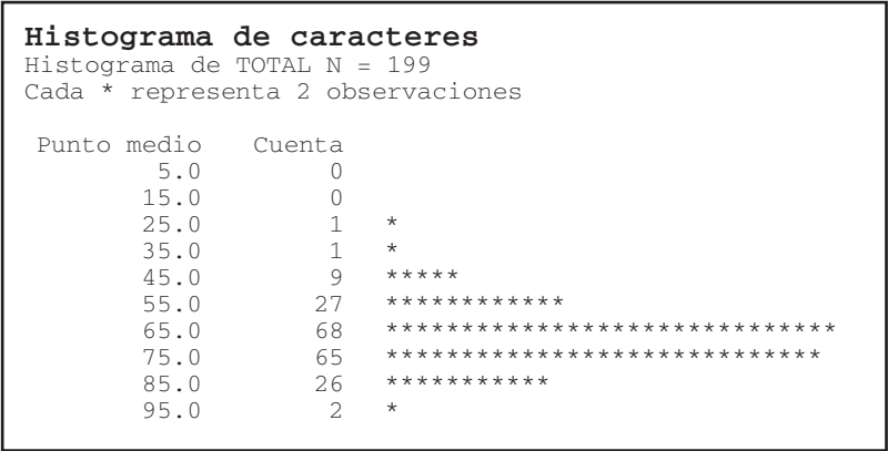
FIGURA 2-15 Histograma y distribución de frecuencias para las calificaciones de Estadística para la administración, obtenidos con Minitab
