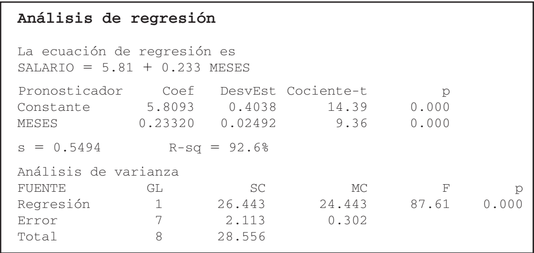
FIGURA 13-10 Regresión con Minitab del salario base sobre los meses de antigüedad
