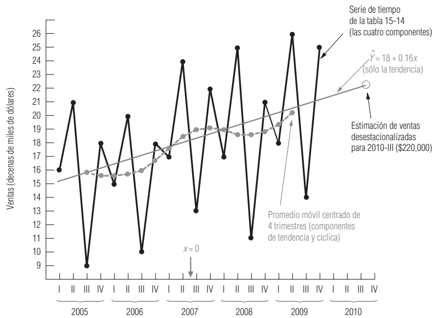
FIGURA 15-8 Serie de tiempo, línea de tendencia y promedio móvil centrado de cuatro trimestres para los datos de ventas trimestrales de la tabla 15-14
