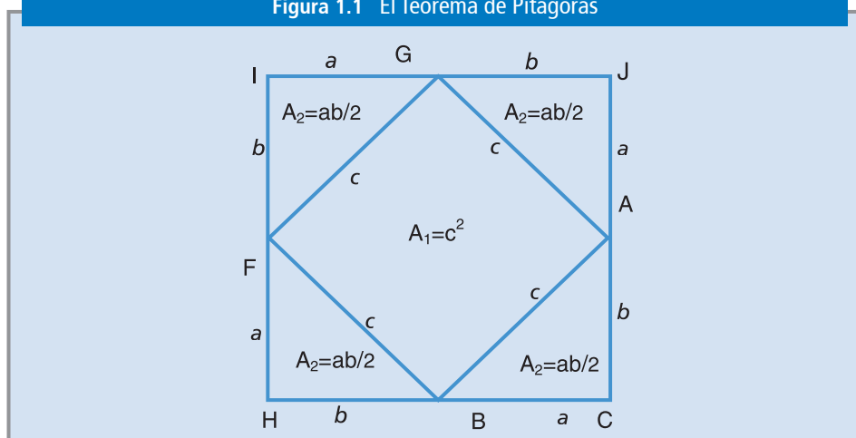
Figura 1.1 El Teorema de Pitágoras
