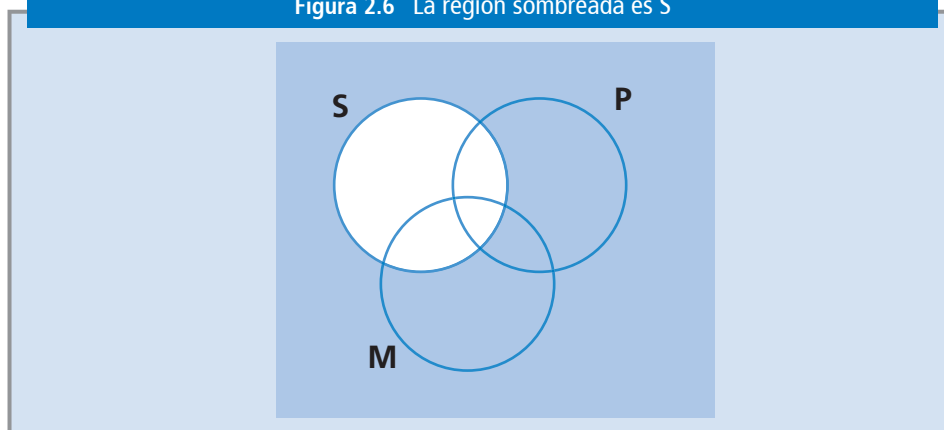
Figura 2.6 La región sombreada es \bar{S}
