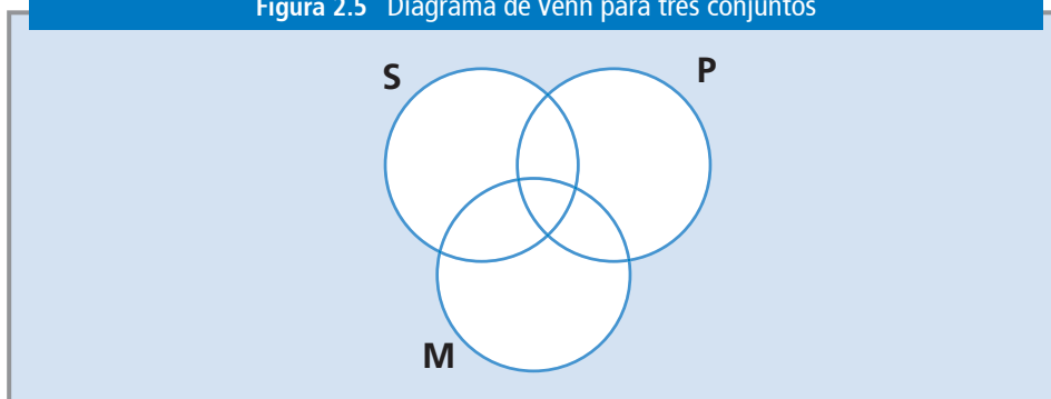
Figura 2.5 Diagrama de Venn para tres conjuntos
