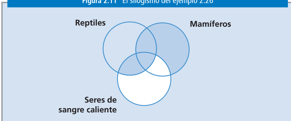
Figura 2.11 El silogismo del ejemplo 2.26
