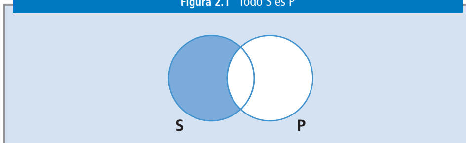
Figura 2.1 Todo S es P
