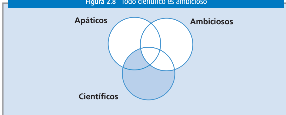
Figura 2.8 Todo científico es ambicioso
