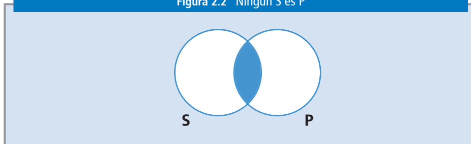
Figura 2.2 Ningún S es P
