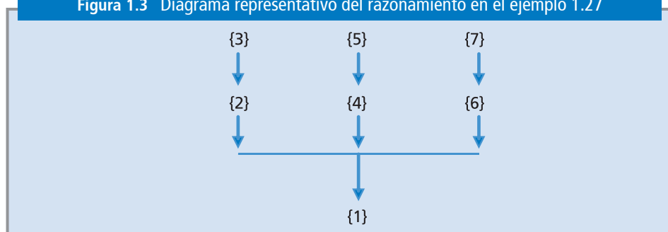
Figura 1.3 Diagrama representativo del razonamiento en el ejemplo 1.27
