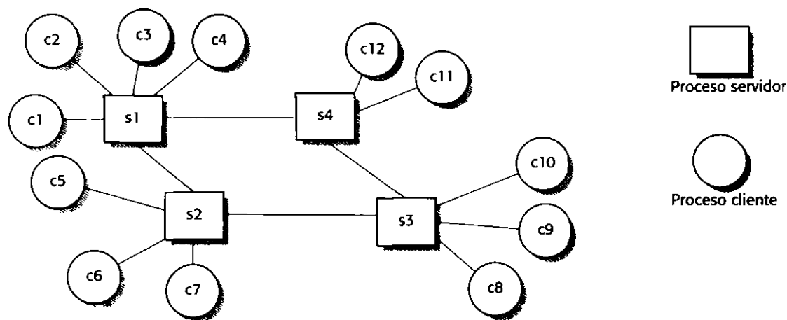
Figura 12.2 Un sistema cliente-servidor.
