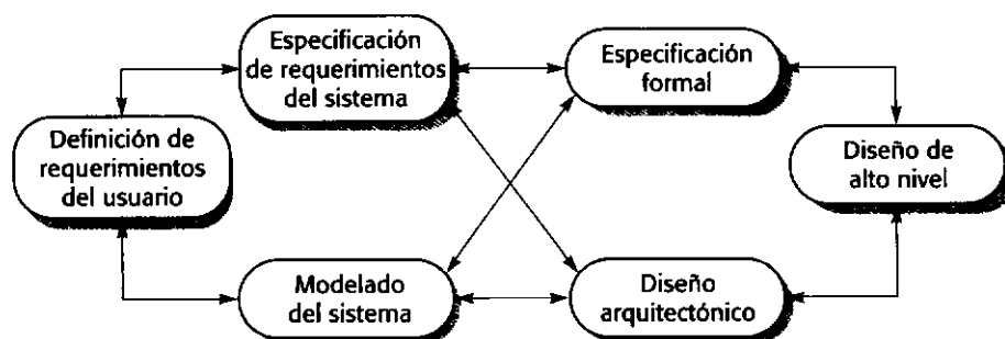
Figura 10.2 Especificación formal en el proceso del software.
