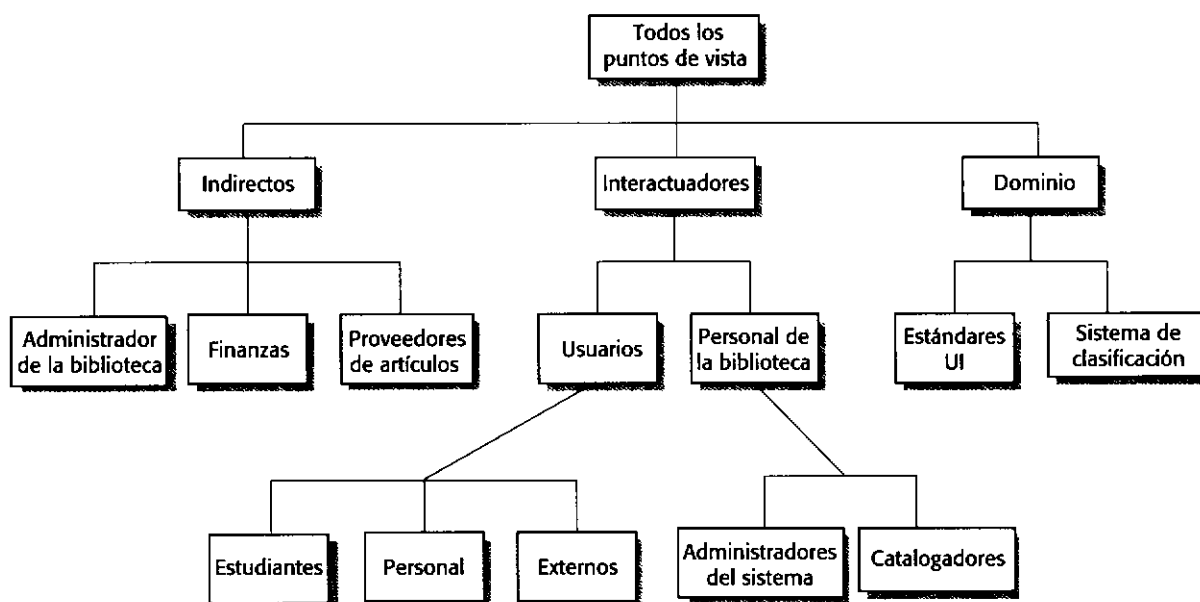
Figura 7.4 Puntos de vista en el LIBSYS.
