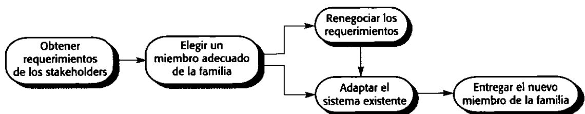
Figura 18.15 Desarrollo de una instancia de un producto.
