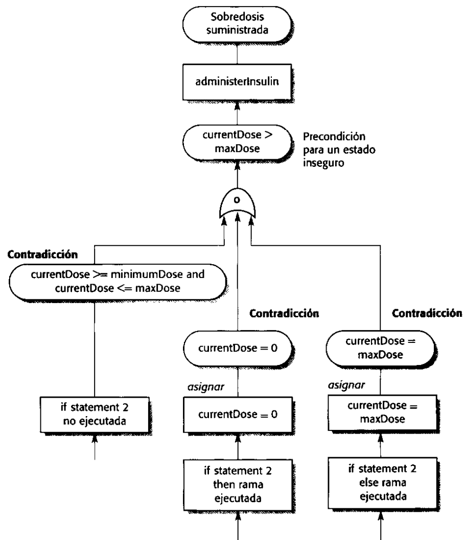
Figura 24.7 Argumento informal de seguridad basado en la demostración de contradicciones.
