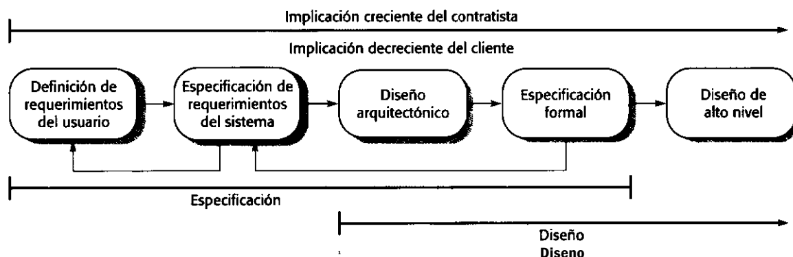
Figura 10.1 Especificación y diseño.
