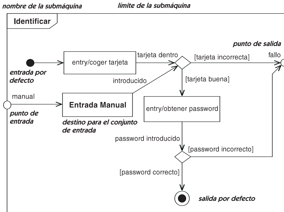
Figura 14.127 Definición de la submáquina
