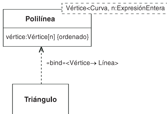
Figura 14.230 Parámetros de clase con restricción
