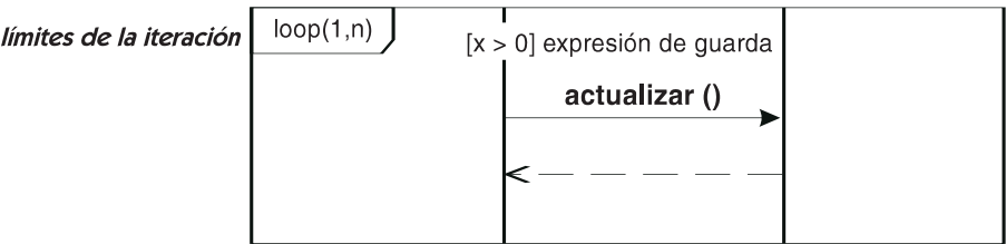
Figura 14.141 Límites de iteración en un bucle
