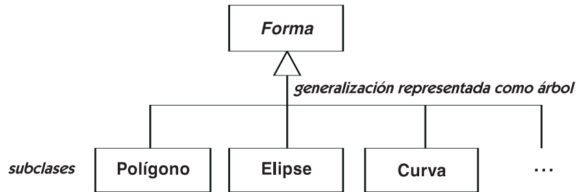
Figura 14.153 Generalización utilizando estilo de árbol
