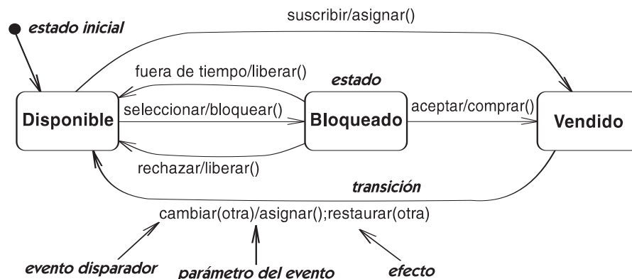
Figura 3.7 Diagrama de máquina de estados de uso
