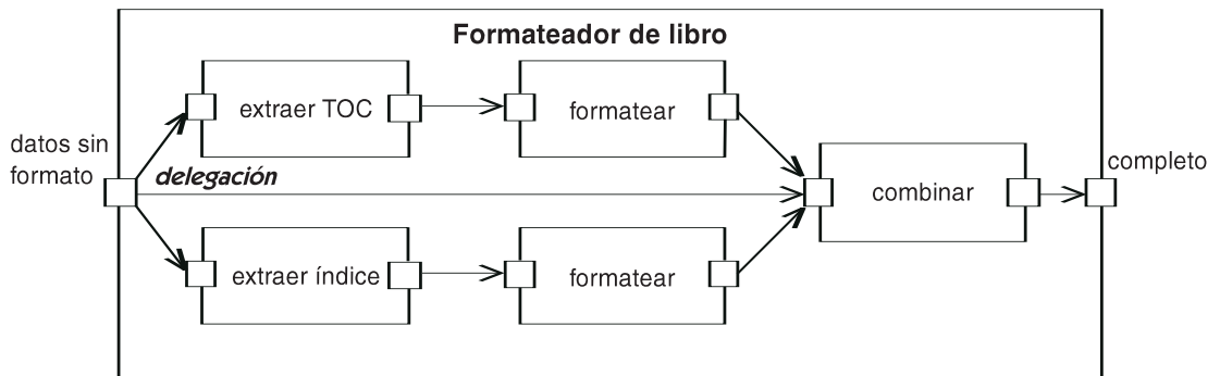
Figura 14.246 Puertos y conectores dentro de una clase estructurada
