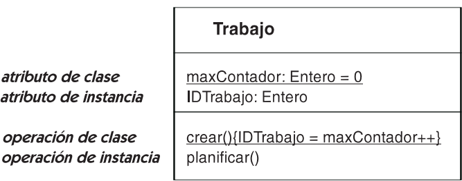
Figura 14.29 Características de clase
