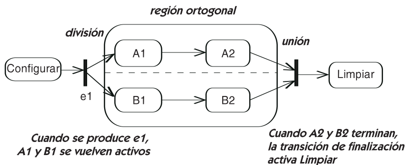
Figura 14.275 División y unión
