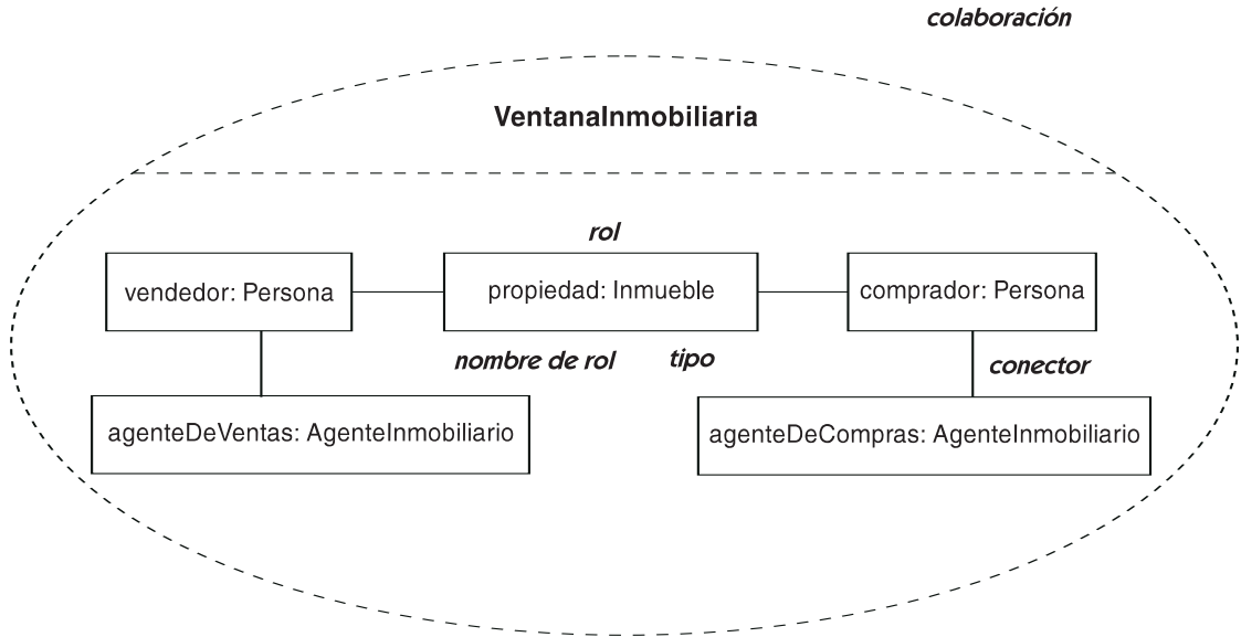
Figura 14.61 Notación de colaboración
