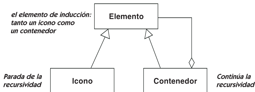
diagrama de clases: recursividad utilizando agregación
