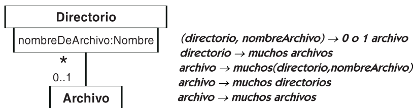
Figura 14.36 Calificador simple
