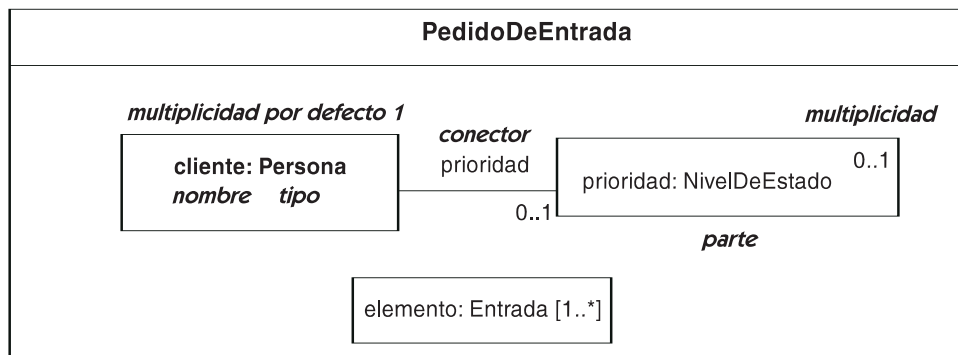
Figura 5.1 Clase estructurada
