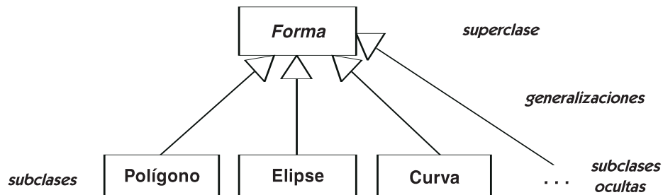
Figura 14.152 Generalización
