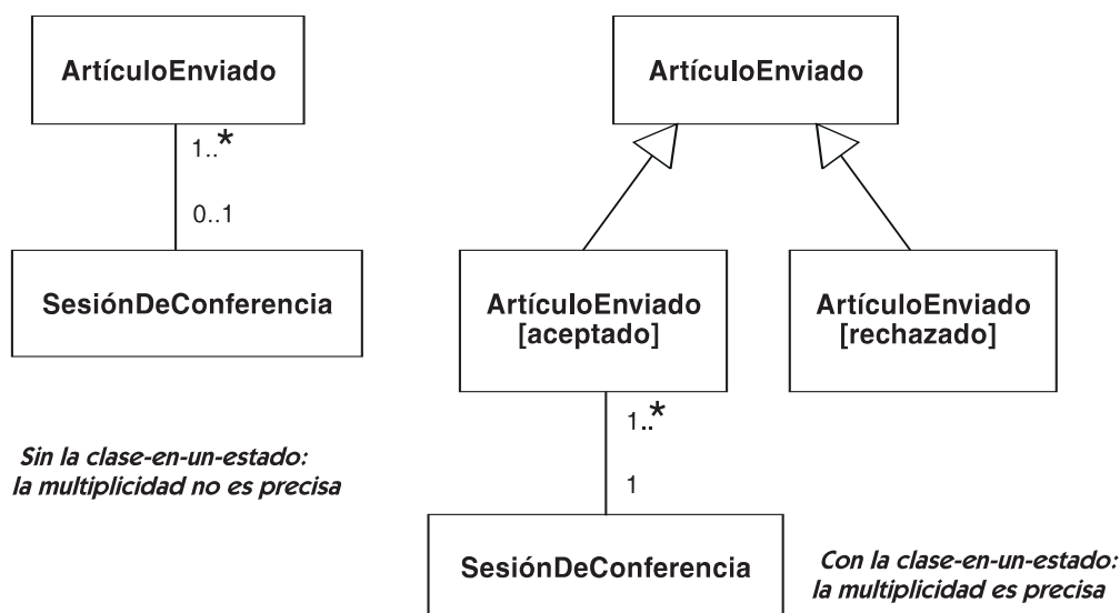
Figura 14.50 Clase-en-un-estado
