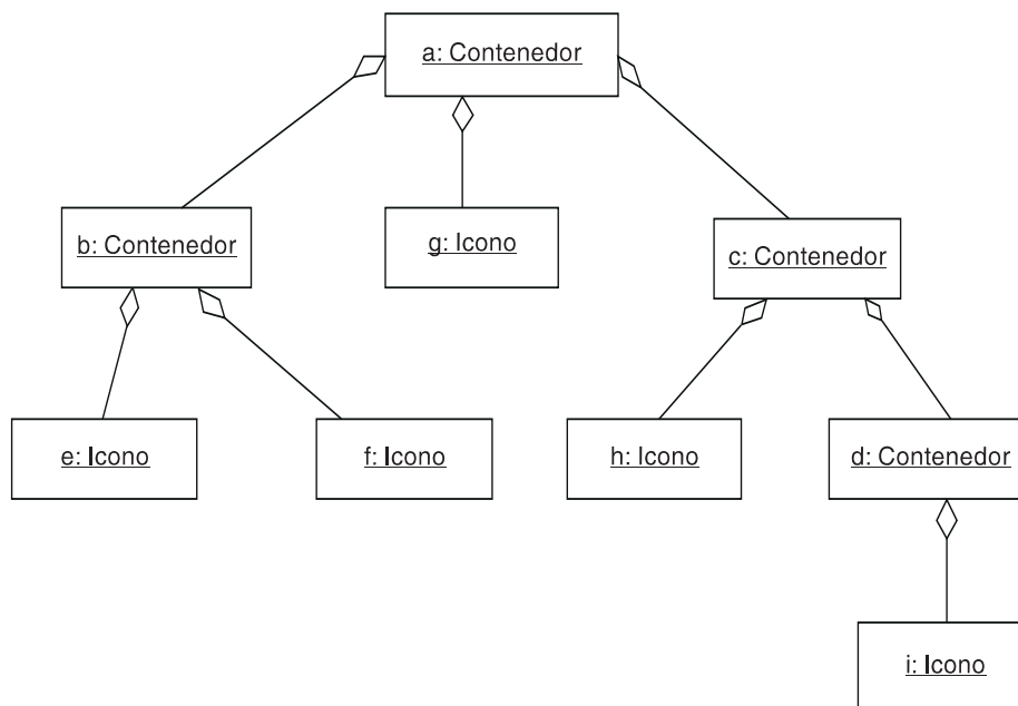
diagrama de objetos: no hay bucles entre objetos
