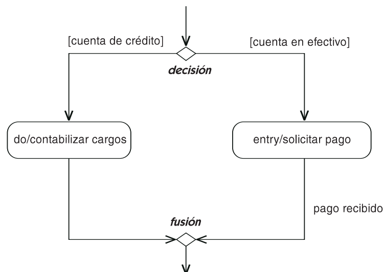
Figura 14.193 Decisión y fusión
