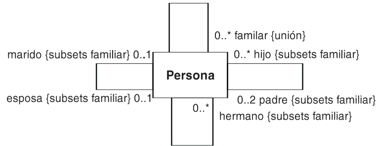
Figura 14.281 Unión derivada
