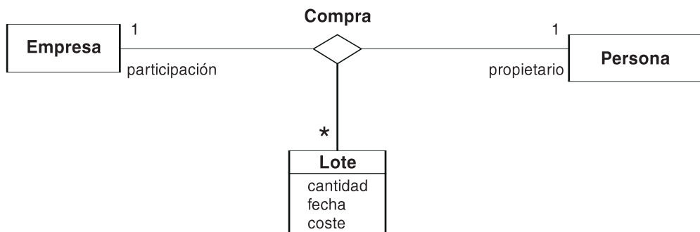
Figura 14.49 Asociación ternaria
