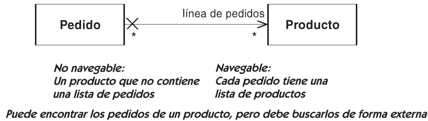
Figura 14.188 Navegabilidad
