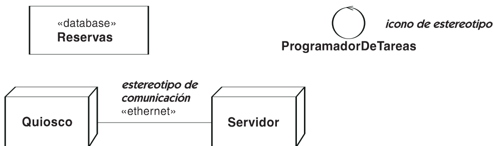
Figura 12.1 Estereotipo
