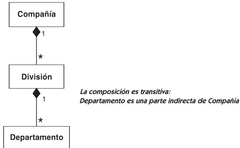
Figura 14.74 Composición multinivel
