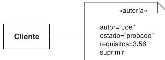
Figura 14.287 Valores etiquetados
