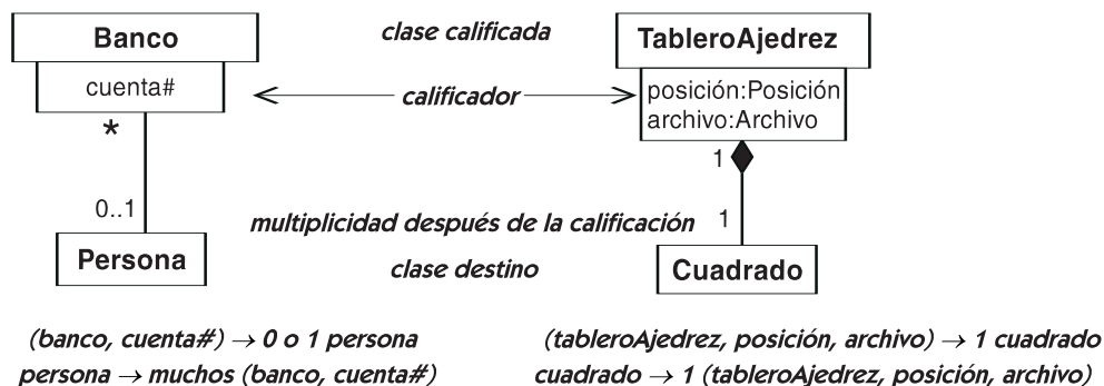
Figura 14.35 Asociación calificada
