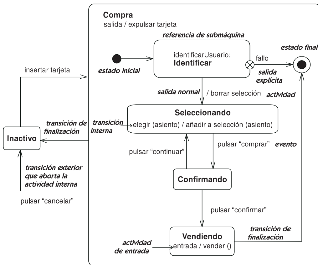
Figura 7.5 Máquina de estados
